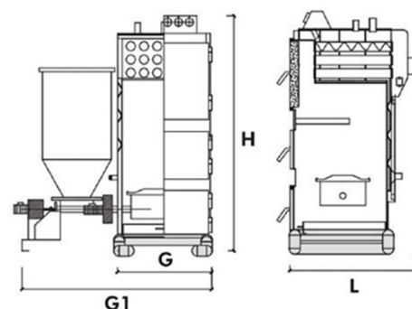
Atmosfere çıkan bacası gazı sıcaklığından maksimum faydayı sağlayan 4 geçişli ve sulubazlı sistem
